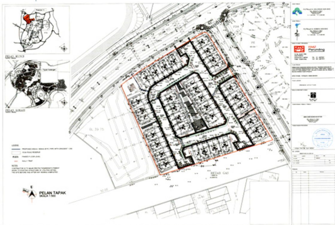
Rajah 4.11 : Pelan Cadangan Jajaran Rangkaian Saliran dan Sistem Perparitan
