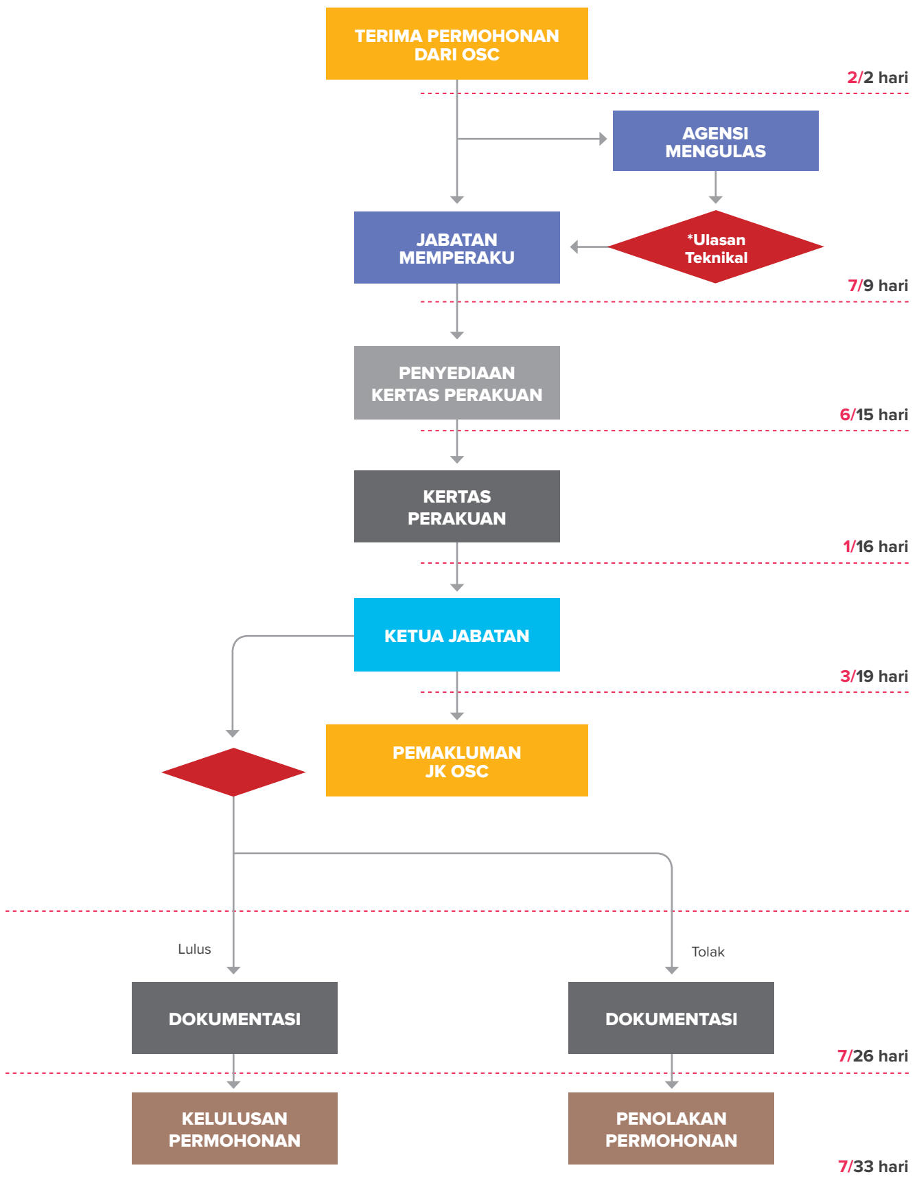
Rajah 6.10 : Carta Alir Kerja Pelan Lampu Jalan/ Nama (Taman, Jalan dan Bangunan) Oleh Ketua Jabatan
